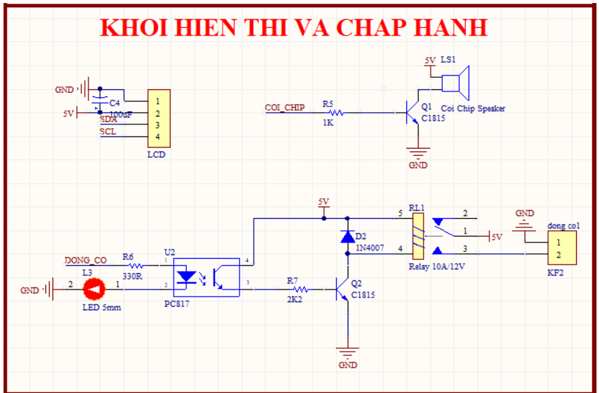
Hình 2.5: Khối cơ cấu chấp hành
